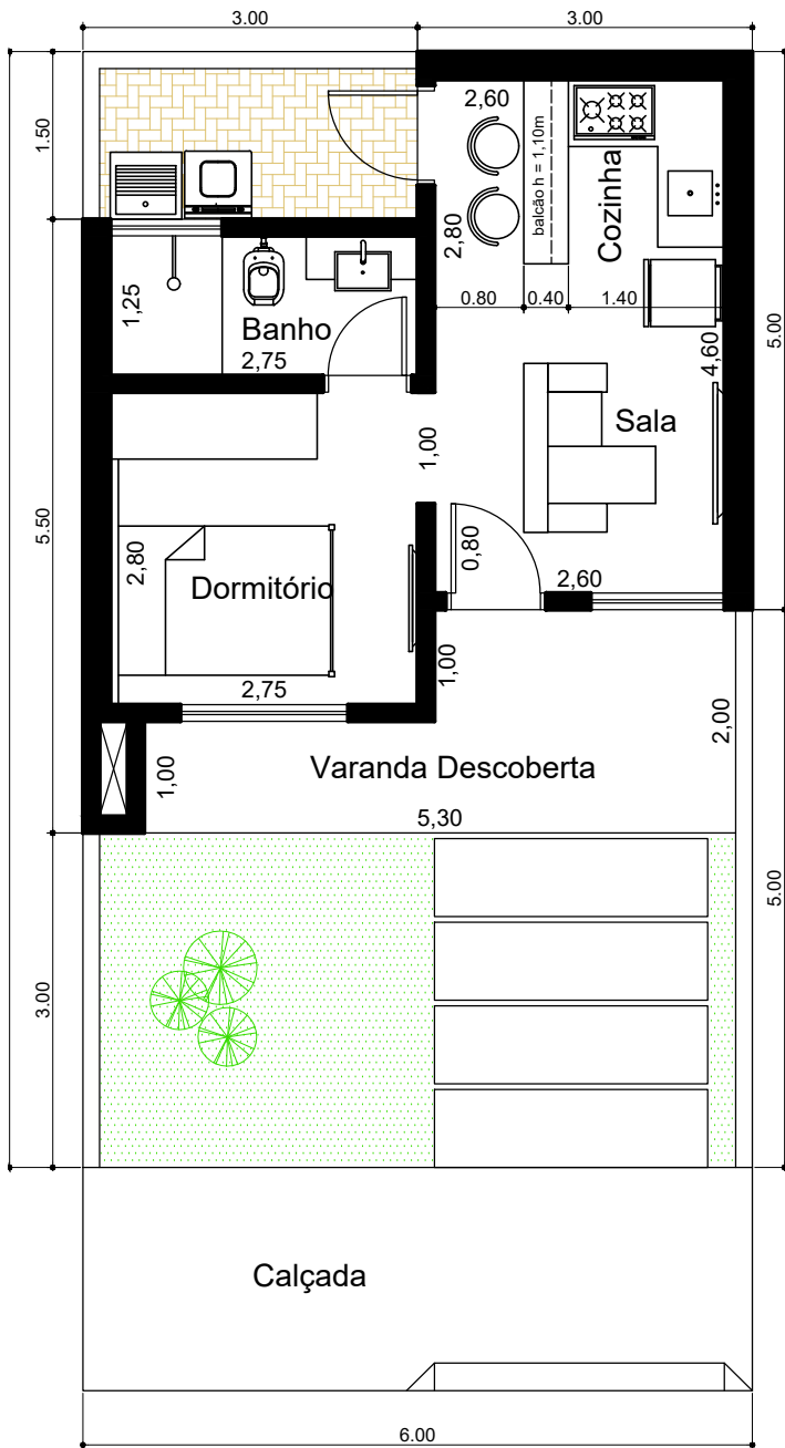
PLANTA CASA 6x10
