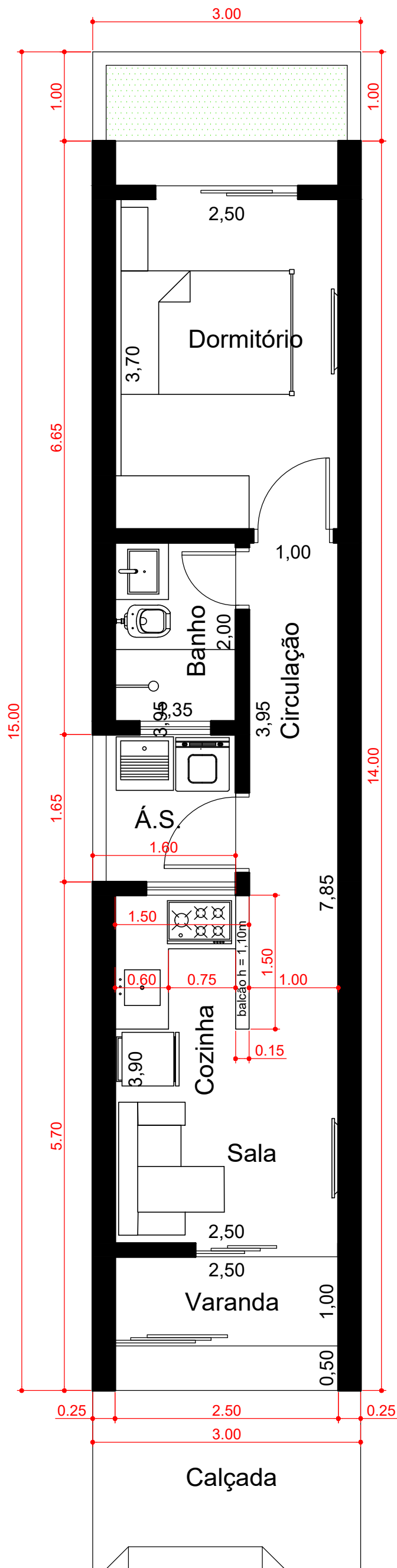
PLANTA CASA 4x15m
