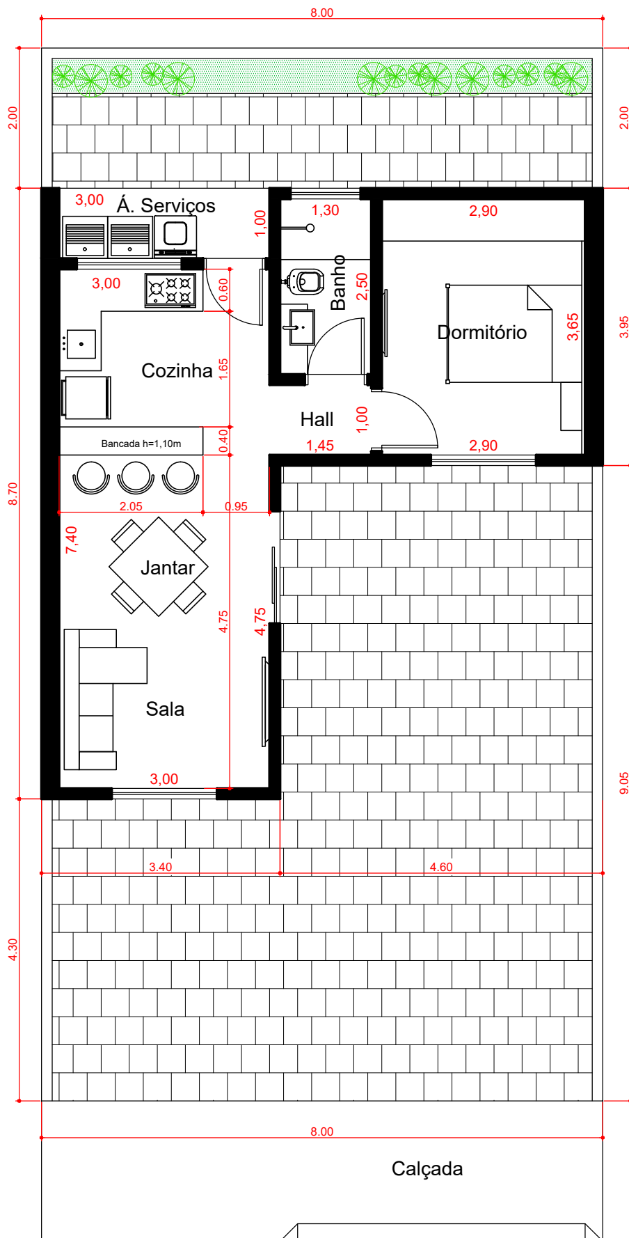
PLANTA CASA EM L 8x15
